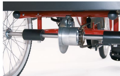
864 Freno a disco applicabile solo sulle versioni con differenziale (207-3D, 4D e 5D).
